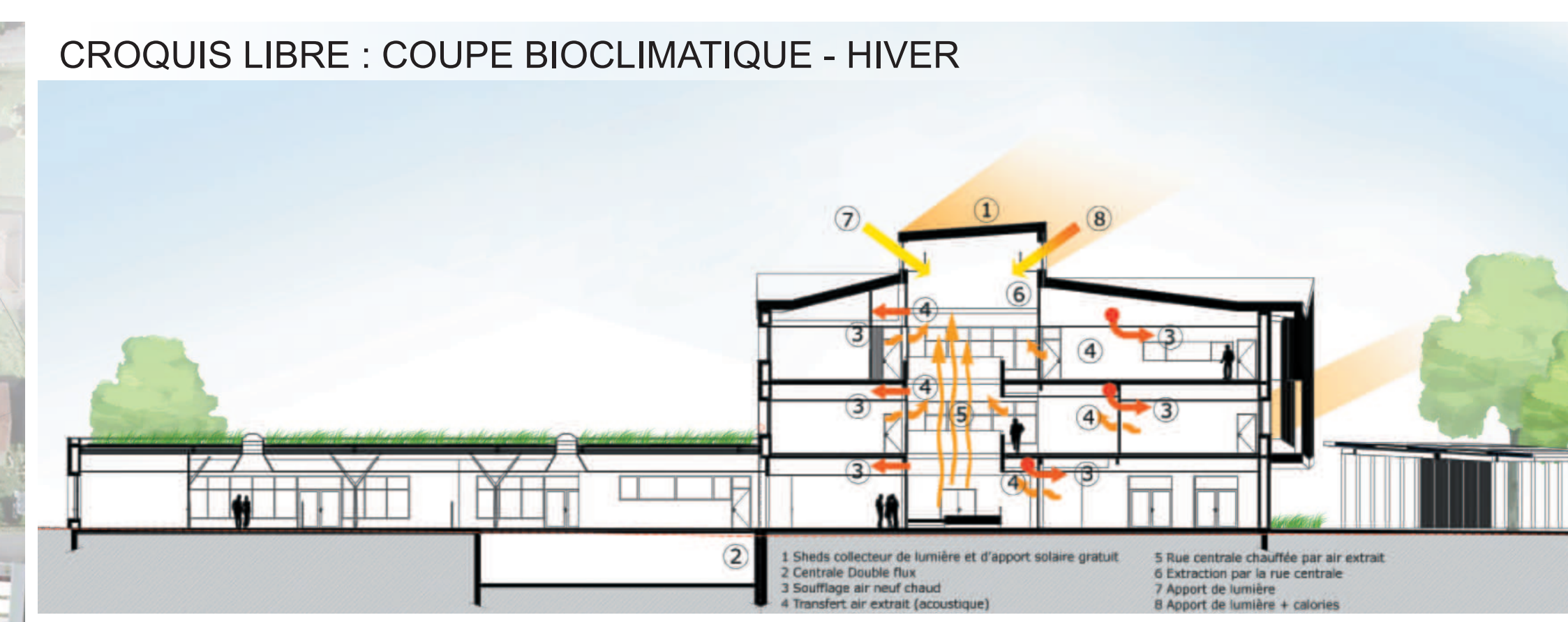
COUPE TRANSVERSALE - 1/200°
