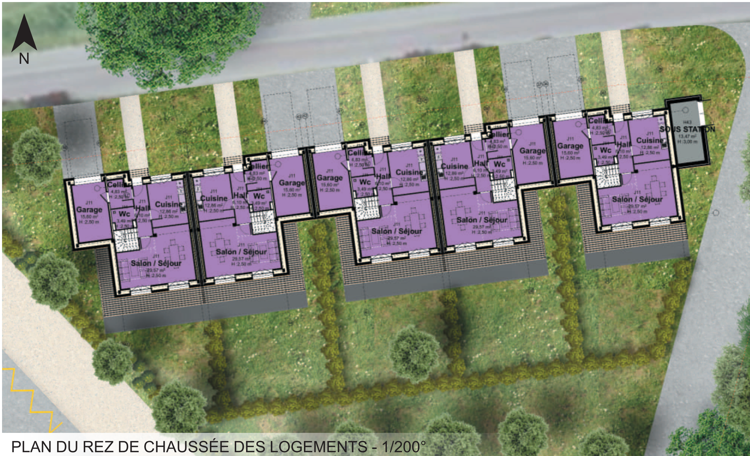
PLAN DU REZ DE CHAUSSEE DES LOGEMENTS - 1/200°
